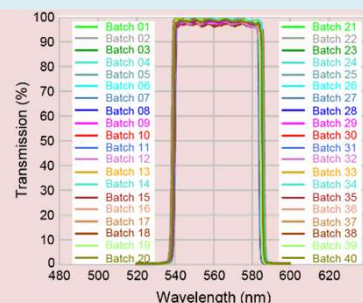
40回分のバッチ間特性比較
